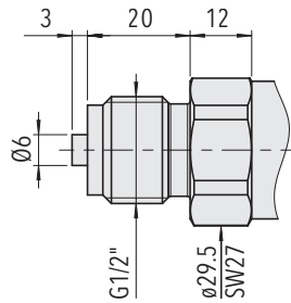
8292.XX.XX11.XX.XX.XX (≤ 600 bar)
