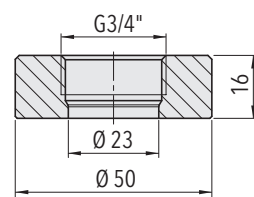
Einschweißflansch für G3/4" Frontmembran (1.4301) Bestell-Nr. C27805
